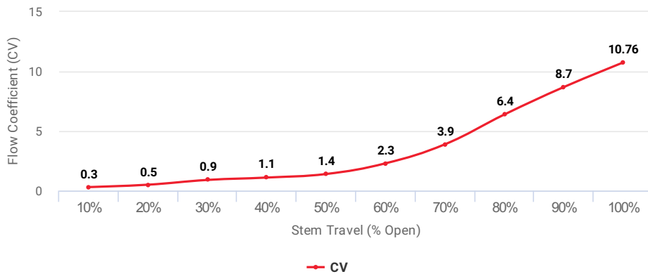
Flow Coefficient (CV) at Stem Travel (% Open) for Item: EEN
